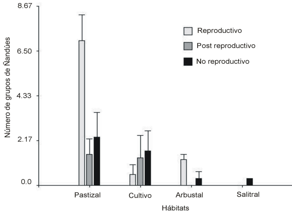
FIG. 1. Número de grupos de Ñandúes (media \pm ES) registrados en los distintos hábitats a lo largo de ciclo anual de esta especie, en el refugio de vida silvestre “Las Dos Hermanas”, Córdoba (Argentina).
